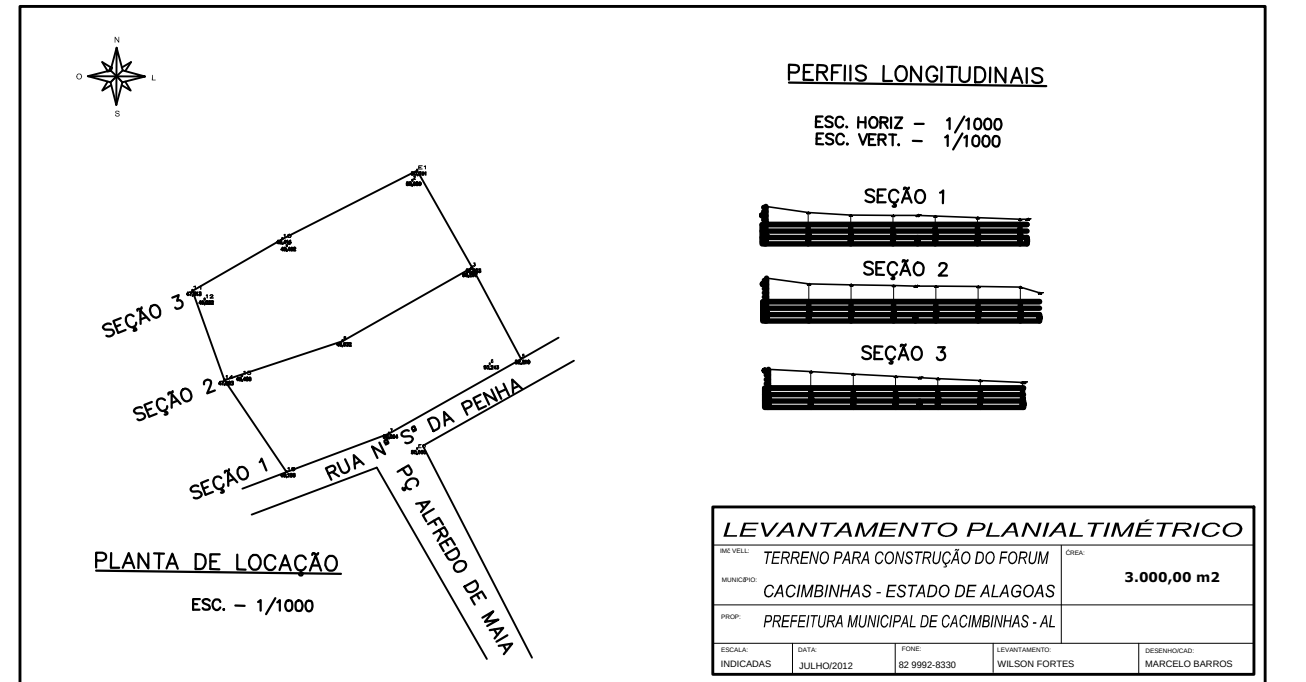
PLANTA SITUAÇÃO
